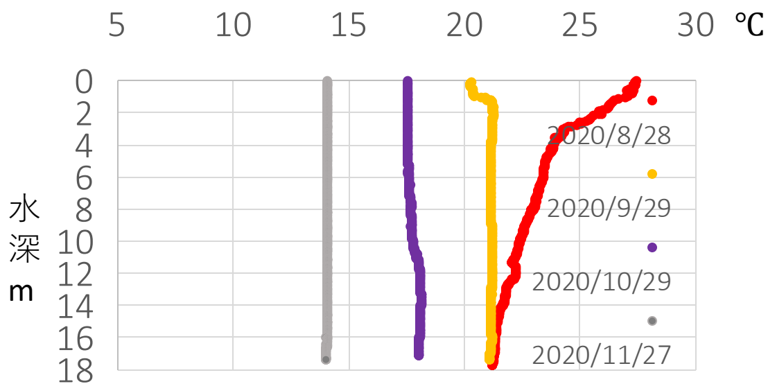
4 カ月ごとの水温変化_2020.8～ (Stn.3)
